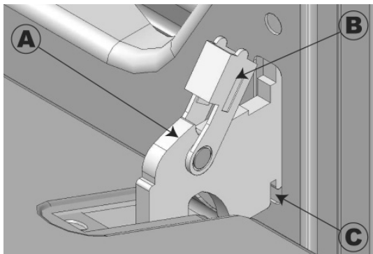
Fig. 4: Bisagra de la puerta del horno
